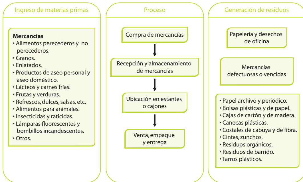
Figura 4. Generación de residuos en el proceso productivo del subsector de minimercados y abarrotes
